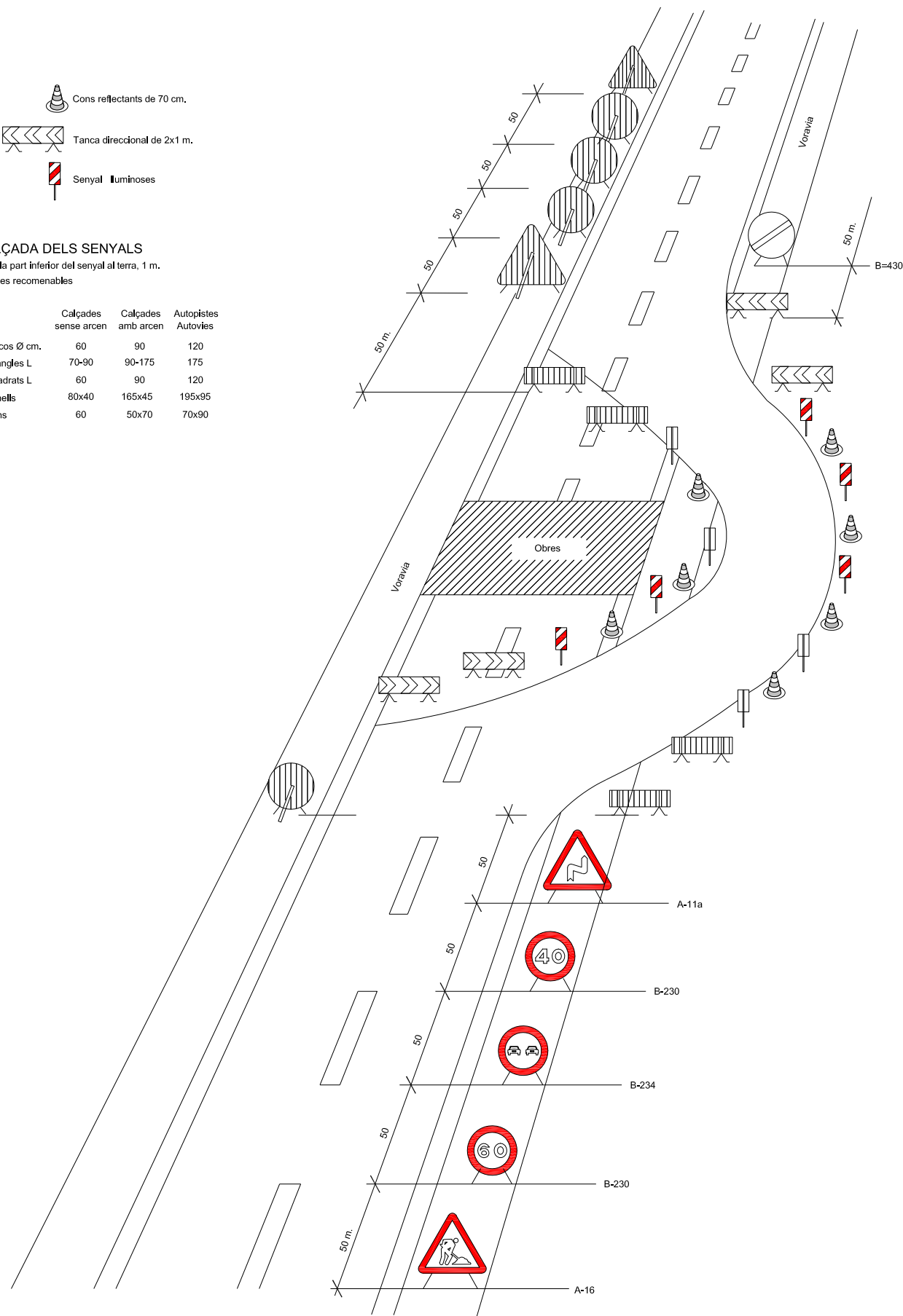
DETALL 010400 Senyalització en talls de carrers amb desviament
