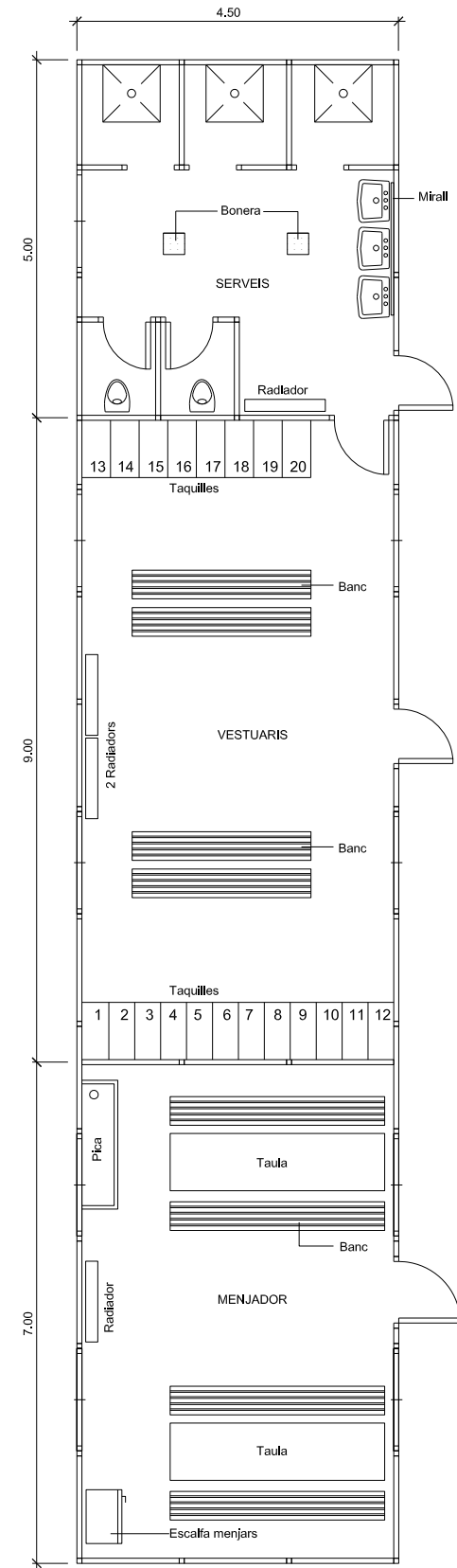
DETALL 020101 Planta barracons tipus ESCALA 1:100
